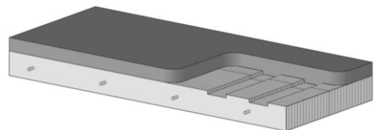
optiholz® Holz-Beton-Verbund
